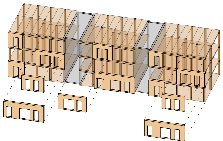
Baukörper C dreigeschossig bestehend aus Modultyp 13
